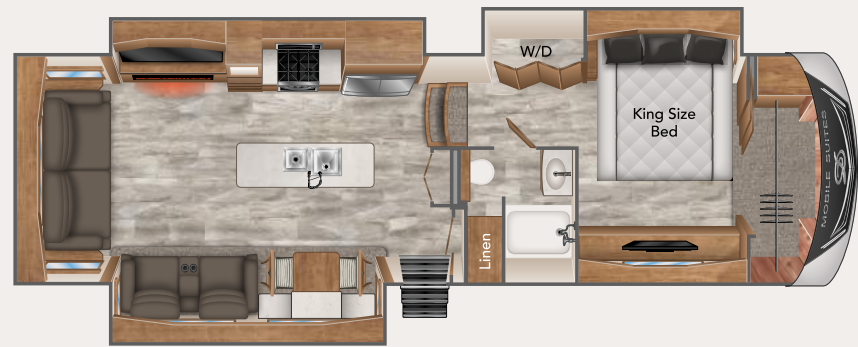
36 RSSB3 Length 36' 9" | Est. Dry 16,600
